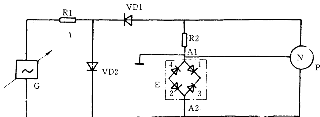
图1 反向重复峰值电流测试电路
